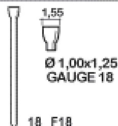
mod. F18
